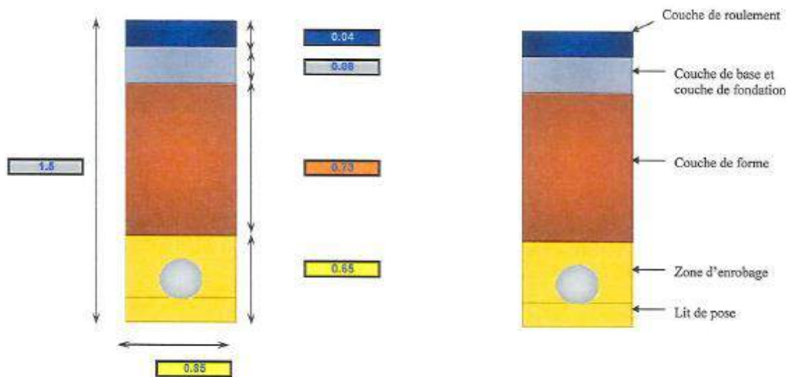
Image 22 : Schéma représentant les caractéristiques de la tranchée
