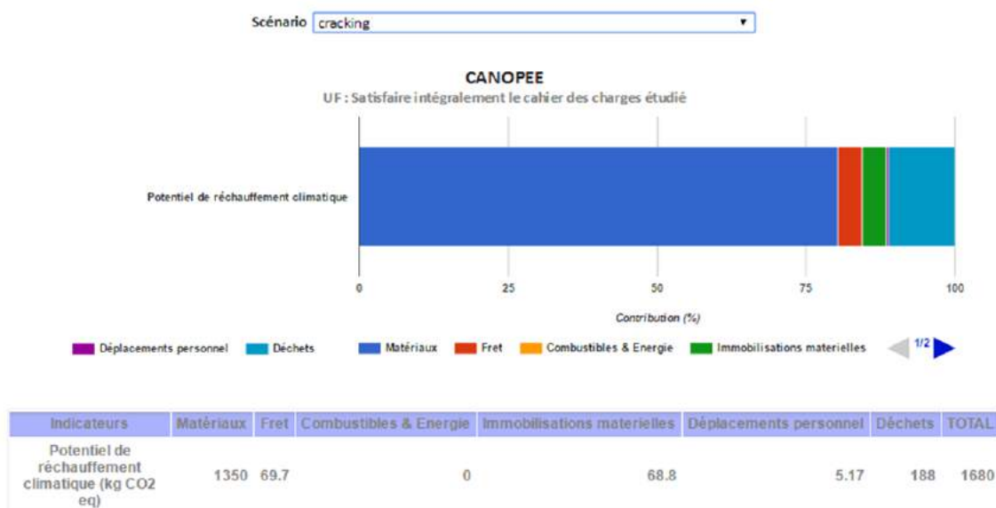
Image 20 : Emission de GES(en kg eq CO2) du chantier par cracking en proportion
