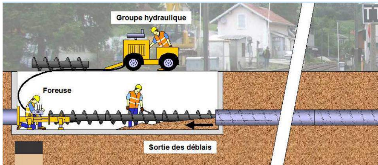
Image 6 : Forage à la tarière [14]
