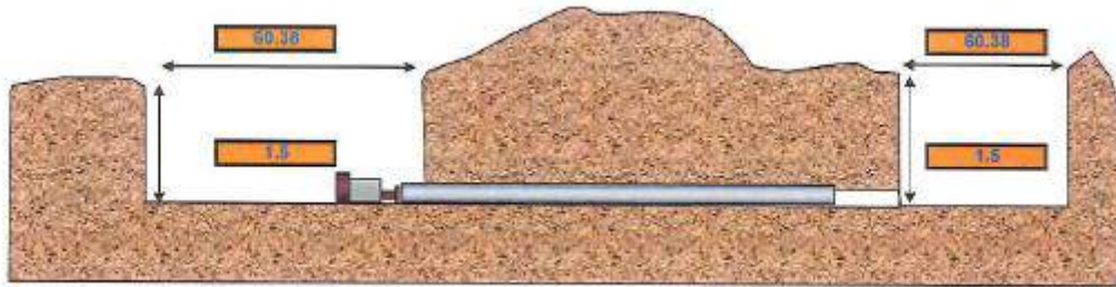
Image 23 : Schéma représentant les caractéristiques des fouilles d'entrée et de sortie pour le cracking
