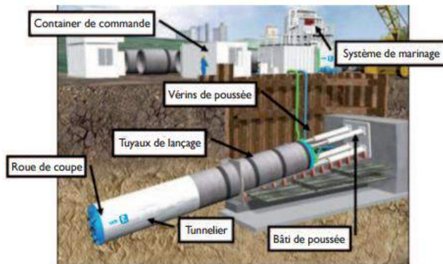
Image 7 : schéma de microtunnelier 5
