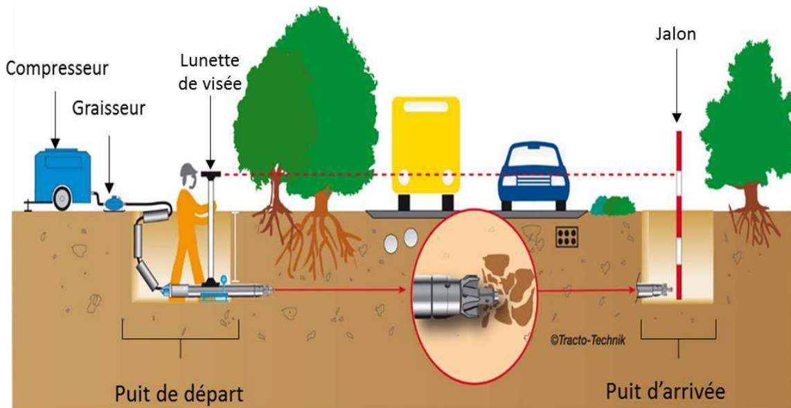
Image 2 : Méthode de forage par fusée pneumatique
