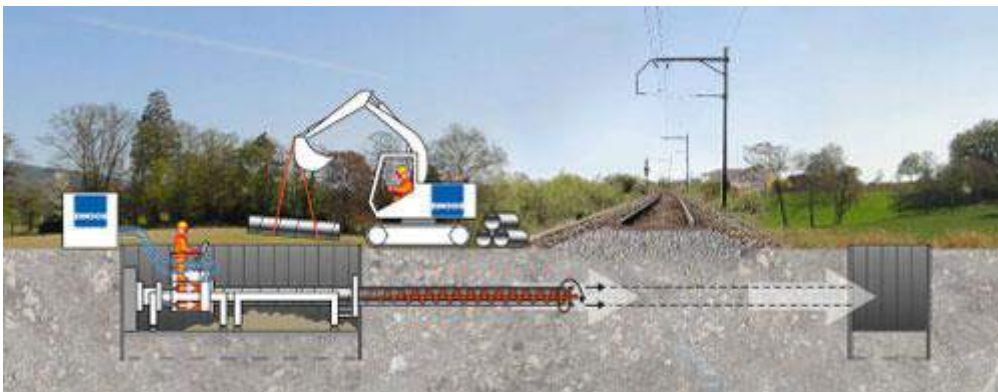
Image 5 : Pousse tube vériné (ou forage horizontal) 4
