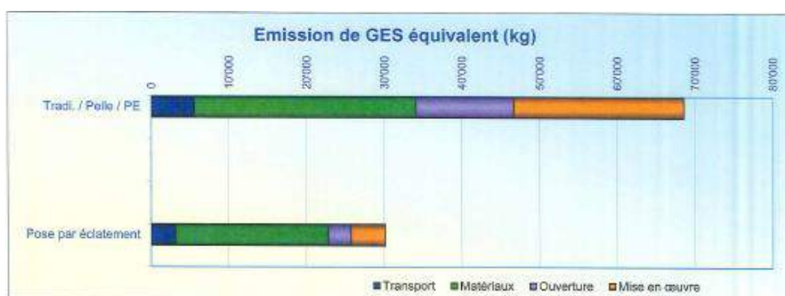
Image 25 : Graphique des émissions de GES du chantier en kg eq. CO2
