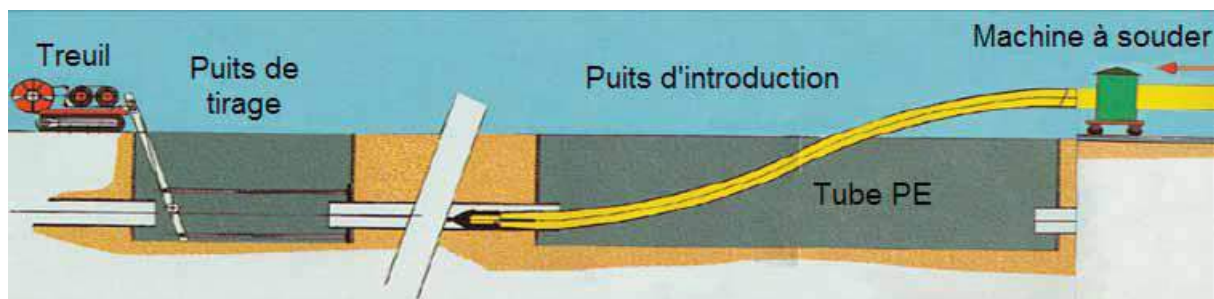
Image 12 : schéma du procédé de tubage simple [22]
