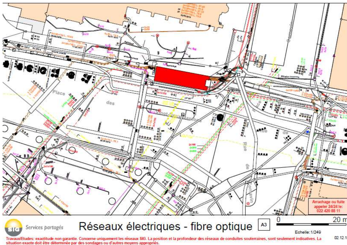
Annexe 1 : Plan des réseaux enterrés électriques – fibre optique, place des 22 cantons à Genève
