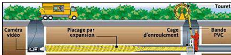
Image 13 : Schéma du procédé de tubage par enroulement hélicoïdal 10
