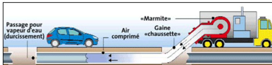
Image 11 : Schéma du procédé de chemisage continu 9
