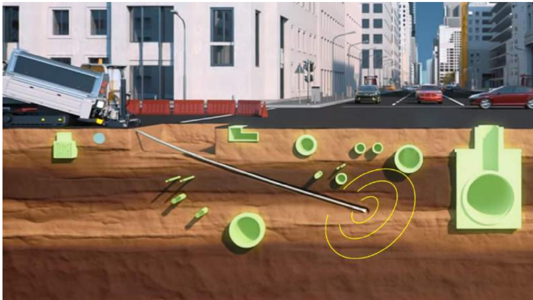
Image 27 : Schéma simplifié du principe de fonctionnement de la technologie ORFEUS 14
