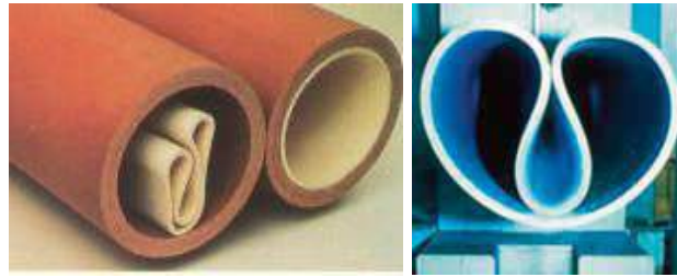
Image 14 : Procédé de tubage par tubes pré-déformés – technique « subline » 11
