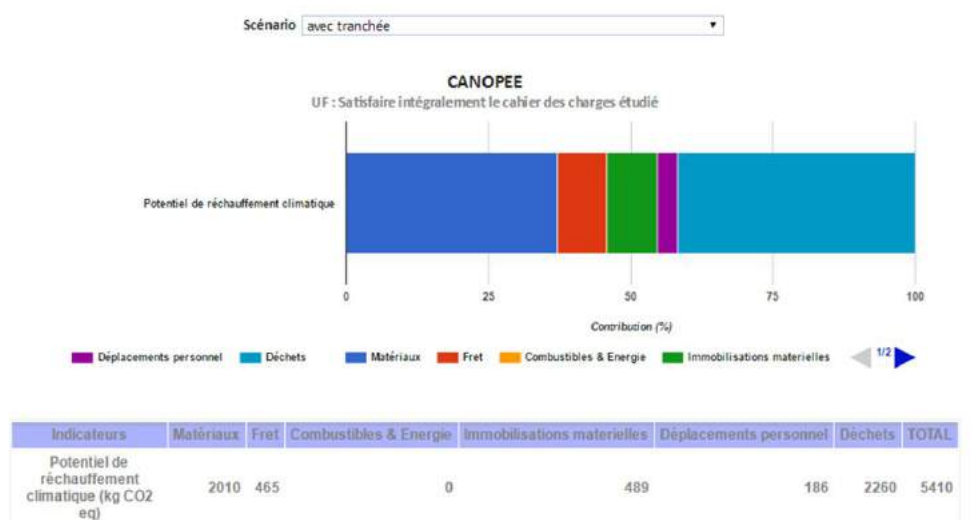
Image 19 : Emission de GES (en kg eq CO2) du chantier avec ouverture de tranchée en proportion
