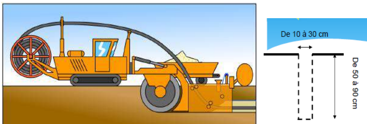
Image 29 : Schéma simplifié de réalisation d'une pose de canalisation par tranchée étroite avec les dimensions associées [33]
