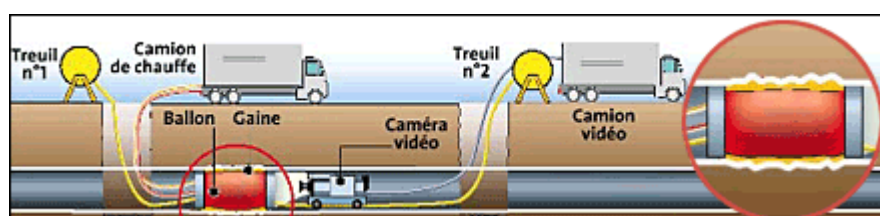
Image 9 : schéma du procédé de chemisage partiel 7
