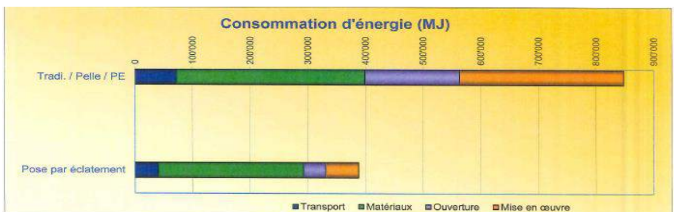
Image 24 : Graphique des consommations énergétiques du chantier en MJ
