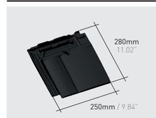
Q102*K | Visum3 left half roof tile klinker
