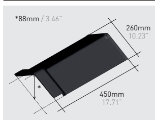
Q110*K | Atica collar ridge klinker
