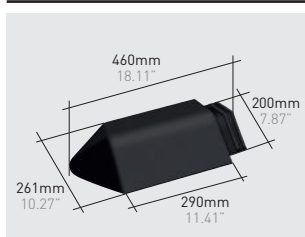
Q109*K | Atica 120° hip / end ridge klinker
