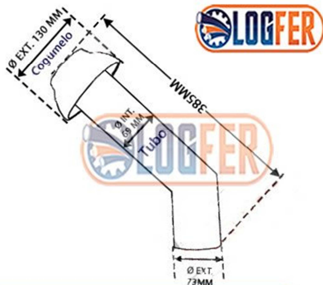
Desenho técnico suporte silo 3"
