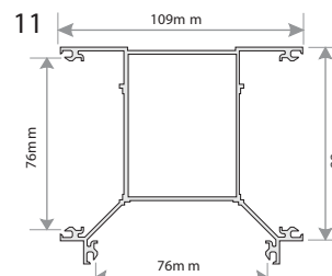
3 Way Box Post Die 6342 (F A 570)
