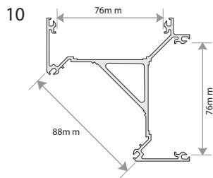
3 Way "Y" Post Die 6343 (F A 580)
