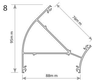
135° / 45° Corner Post Die 6324 (F A 550)
